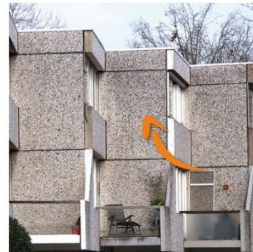
Gevelisolatie zijgevel: Rc 1,5
